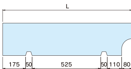
● 正面図
