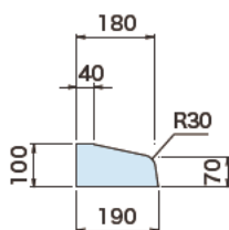
●断面図
