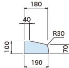
●断面図
